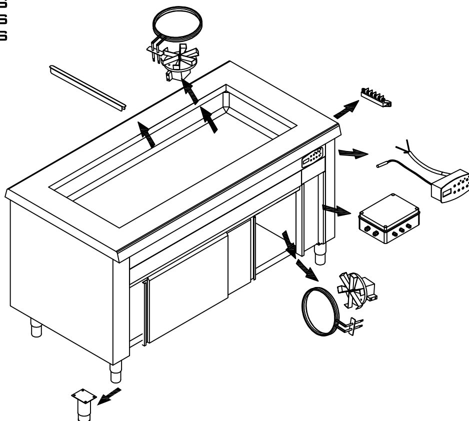
VENTILATEUR EMB POUR CUVE A' AIR COD.30480006
