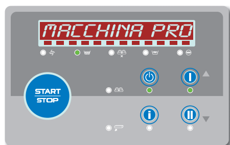
Exemple de machine prête avec alarme en cours
